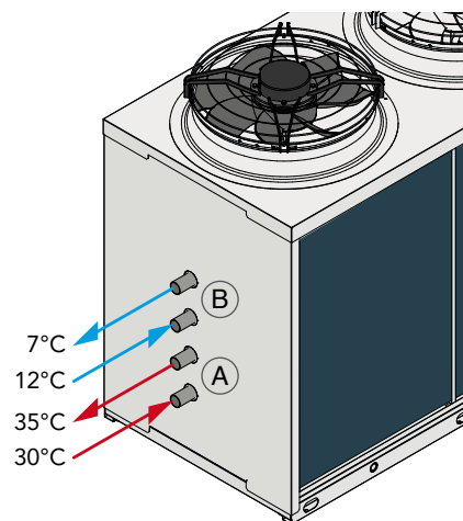
Gleichzeitiger Kühl- und Heizbetrieb
