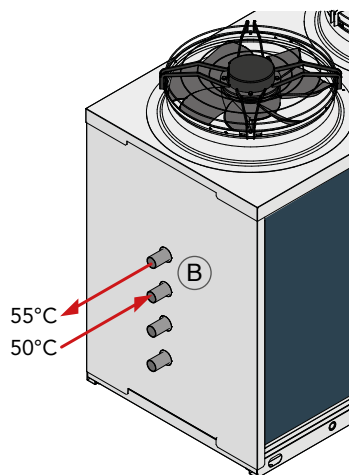
Warmwasserproduktion
