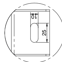
DETTAGLIO A
