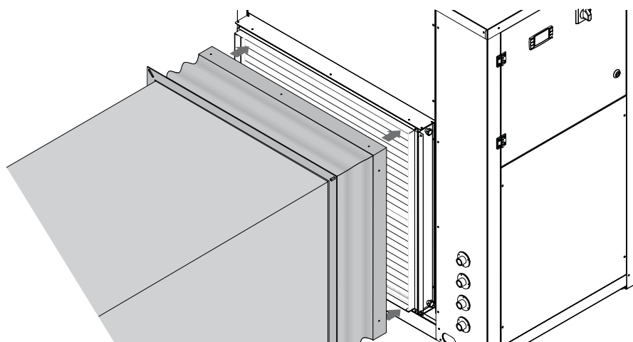
Fixage du canal au bouches de soufflage et reprise
