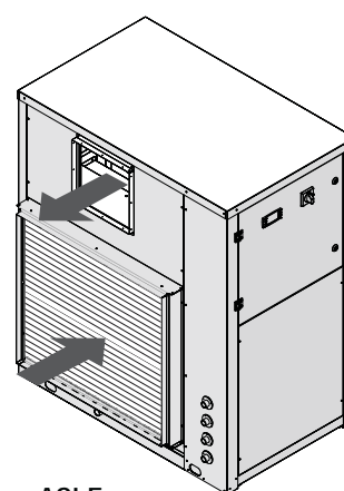
ASLE Impulsión horizontal derecha
