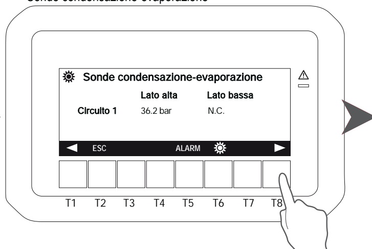
Sonde condensazione-evaporazione
