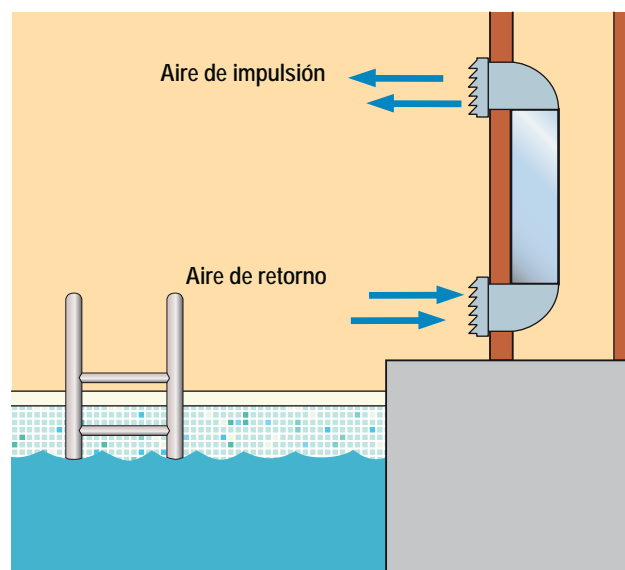
Instalación versión canalizada P con plenum de impulsión y retorno a 90°
