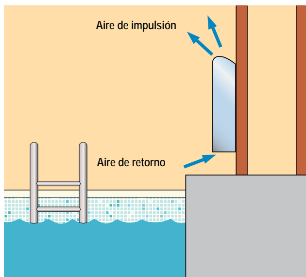
Instalación versión estándar A
