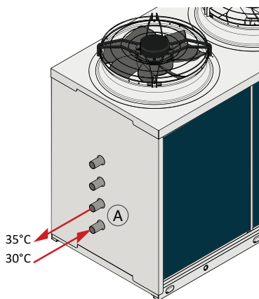
Verbraucher- Heizung
