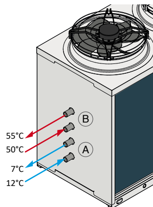
Refrigeración por agua instalación + Calefacción A.C.S.
