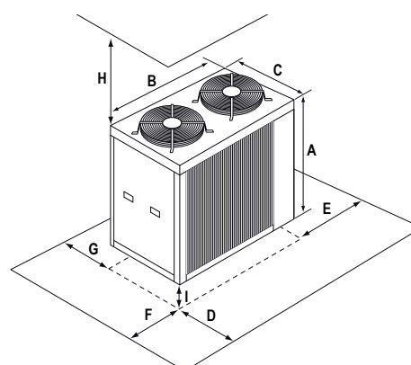
Unità esterna
