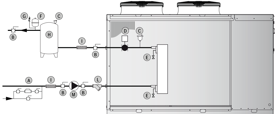
Circuito instalación
