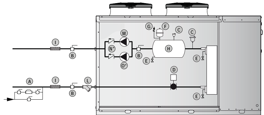
Circuito instalación
