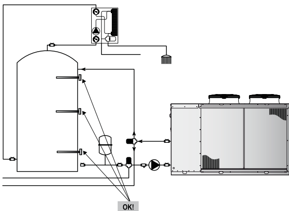
Richtige Positionierung des BTS-Sensors
