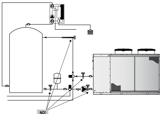
Falsche Positionierung des BTS-Sensors
