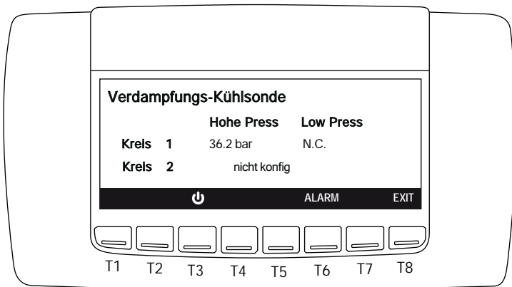
Sensoren Druckanzeige
